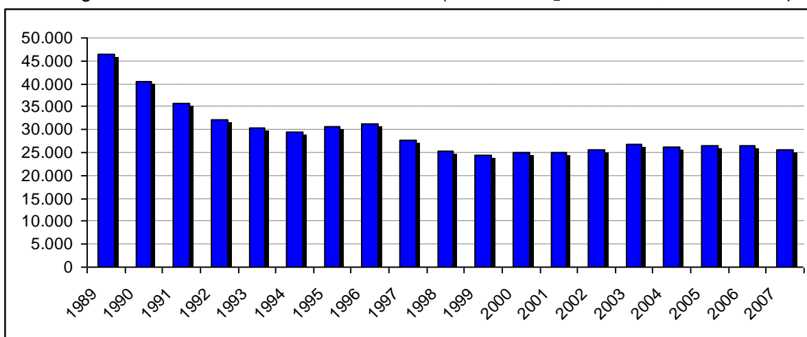
Figura 3.4.1. Nivelurile emisiilor de metan (mii tone CO 2 echivalent, fără LULUCF)
